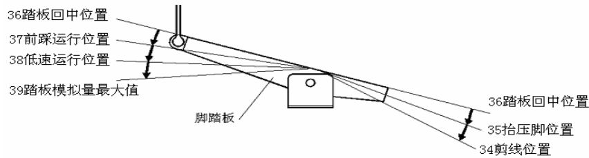
图 2-1 踏板动作参数各位置示意图
